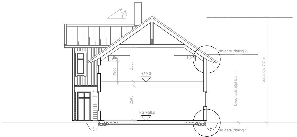
SEKTION A-A 1:100
